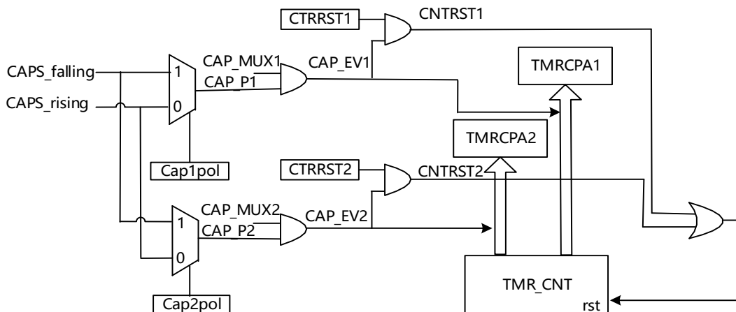
图 15-3 输入捕获模式框图
