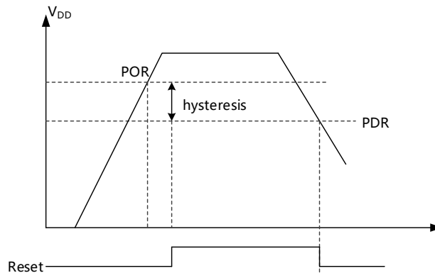
图 8-1 上下电复位波形图
