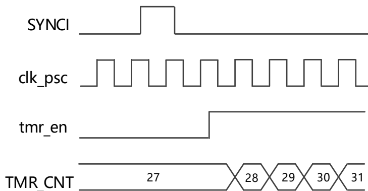
图 15-5 TIMER 触发模式波形图
