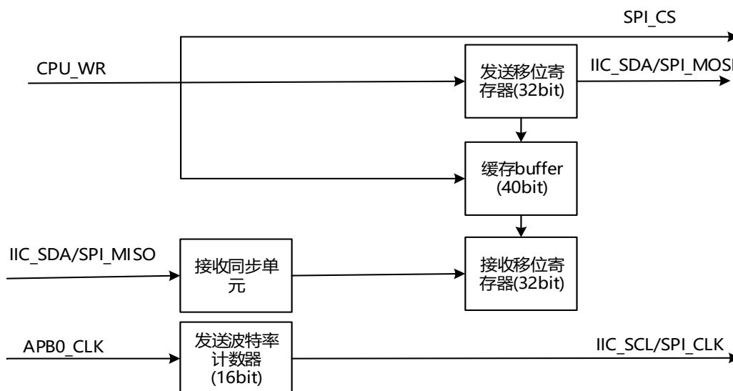
图 12-1 SPI/IIC 模块架构图
